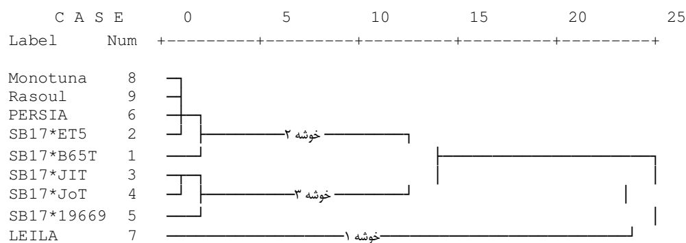
شکل ۱ تجزیه خوشه‌ای بر مبنای صفات عملکردی و کیفی هیبریدها در منطقه کرج طی سال‌های ۱۳۸۶-۱۳۸۷
