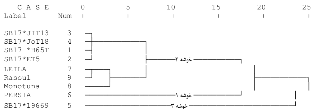
شکل ۲ تجزیه خوشه‌ای بر مبنای صفات عملکردی و کیفی هیبریدها در منطقه دزفول طی سال‌های ۱۳۸۶-۱۳۸۷
