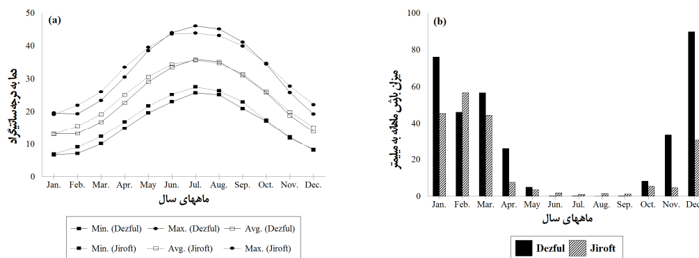
شکل ۱ تغییرات میانگین بلندمدت ماهانه (a) حداقل، متوسط و حداکثر دما و (b) میانگین بارش ماهانه مناطق دزفول و جیرفت
